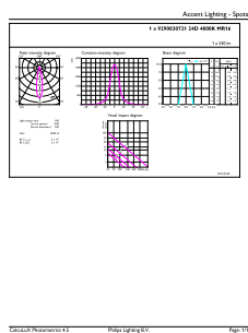
LEDspots GMGC 1 6,5W MR16 GU5,3 940 24D-ADL
